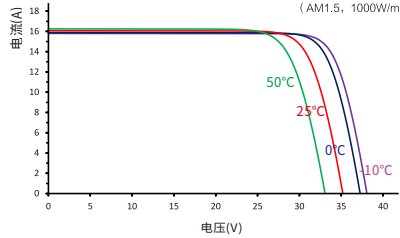
不同电池温度下, I-V 曲线图
