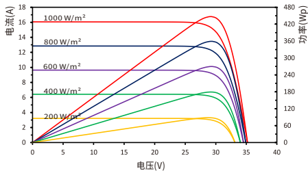
不同辐照度下, I-V 曲线图
