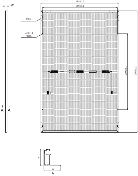
产品图示 单位: mm
